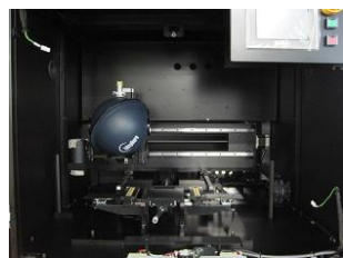
LEDボード用 半自動測定機
